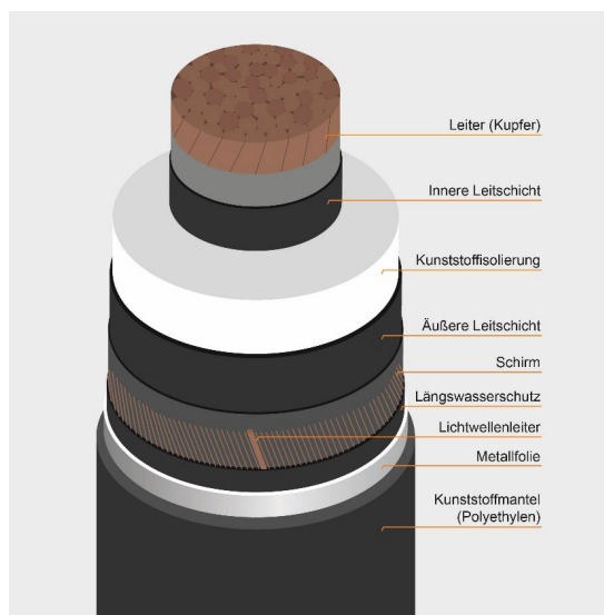
Querschnitt eines Erdkabels
