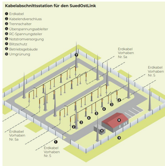
Schematische Darstellung einer Kabelabschnittsstation (KAS) für zweimal zwei Gigawatt.
