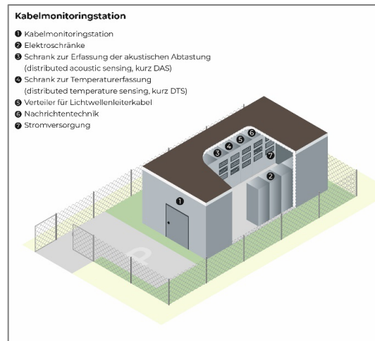
Schematische Darstellung einer Kabelmonitoringstation für 2 Gigawatt
