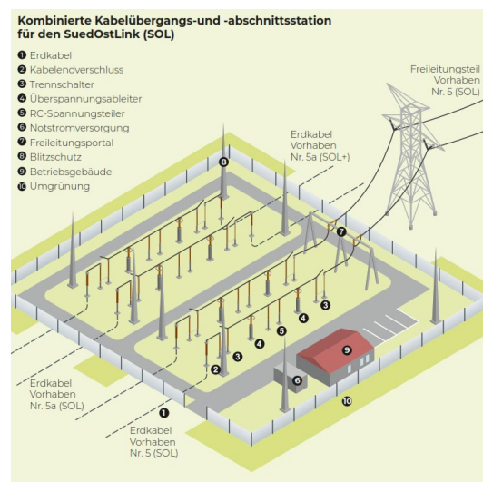
Schematische Darstellung einer kombinierten Kabelübergangs- und -abschnittsstation
