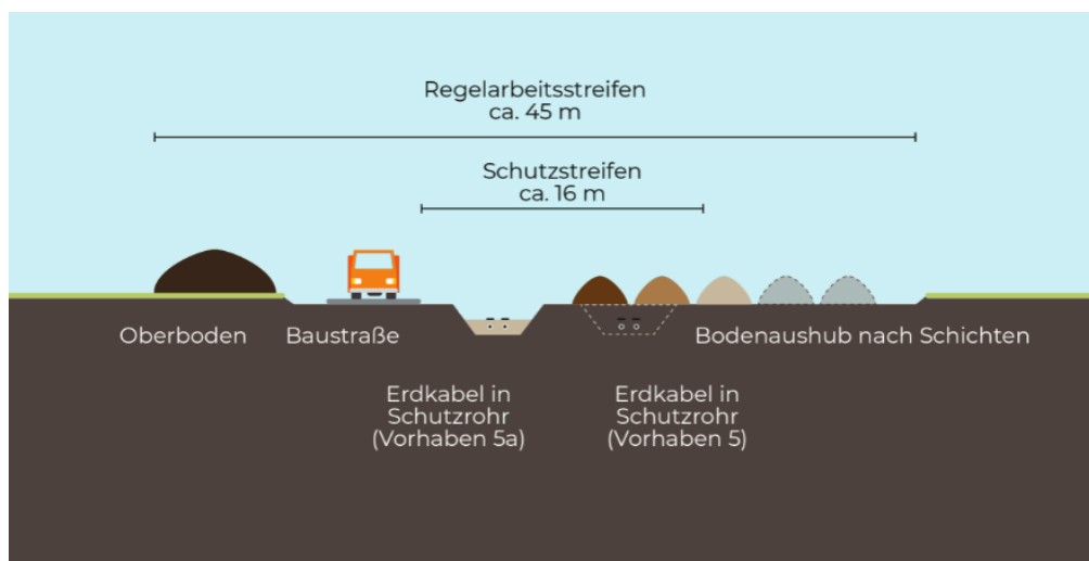
Baustelle für Erdkabel mit zwei Kabelgräben im Offenland
