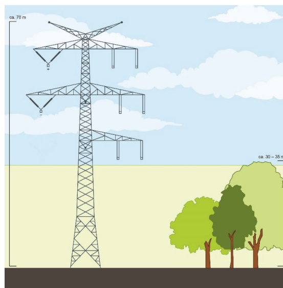
Beispiel für Hybridmast für 525 Kilovolt (kV) Gleich- und 380 kV Wechselstrom
